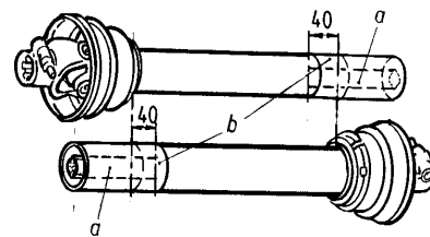
Bild 6. Förkortning av kraftöverföringsaxel
